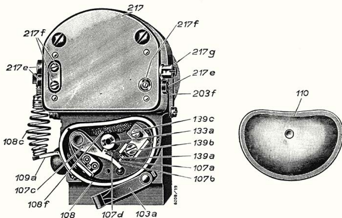
103 a = Deckelhalter 133 a = Nocken 107 a = Amboßkontakt 139 a = Amboß 107 b = Hebelkontakt 139 b = Klemmschraube zum Befestigen des Ambosses 107 c = Unterbrecherhebel 139 c = Verstellerschraube 107 d = Gleitstück im Unterbrecherhebel 203 f = Deckplatte 108 = Unterbrechergehäuse 217 = Reglerschutzkapsel 108 c = Rückzugfeder 217 e = Gummitüllen 108 f = Filz für Nockenschmierung 217 f = Anschlußschrauben 109 a = Verstellhebel 217 g = Umschalter 110 = Unterbrecherdeckel
