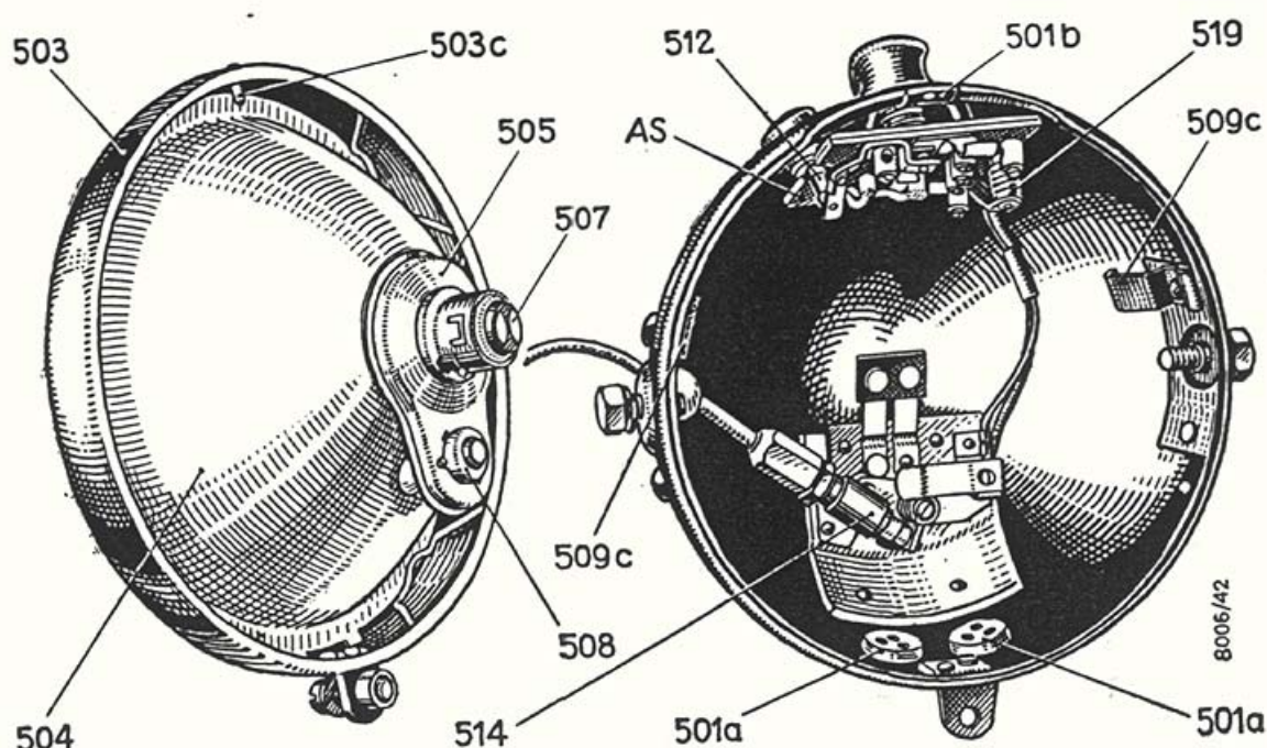
Bild 12 Scheinwerfer, geöffnet
