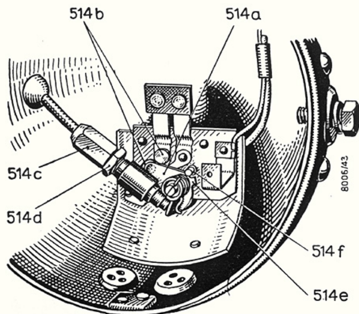
Bild 14 Abblendumschalter
