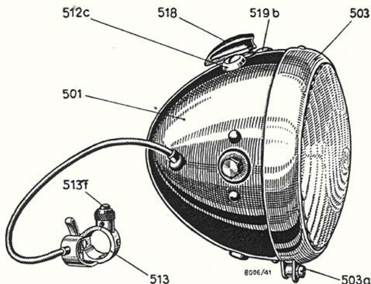
Bild 11 Scheinwerfer EAS 150x2
