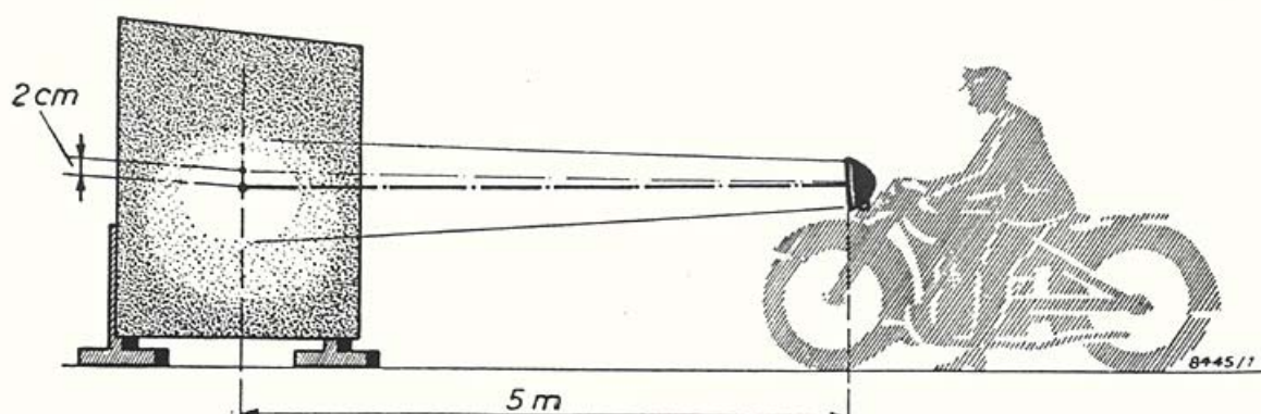
Bild 13 Einstellen des Scheinwerfers
